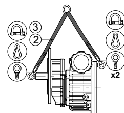
VR 3 - VR 5.5
