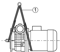
V 0.5 ... V 10
